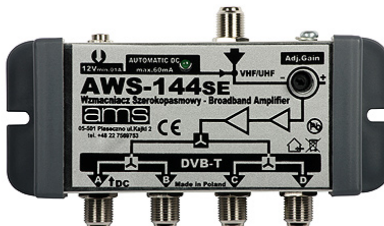
Widok wzmacniacza z góry
