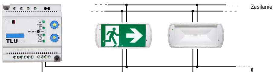
TLU (LUM10312)
