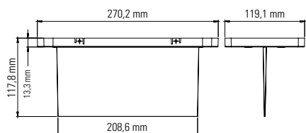
Klosz SL2PP
