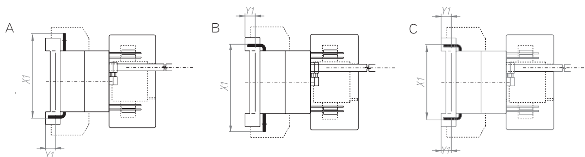
Niestandardowe zaciski przyłączeniowe
