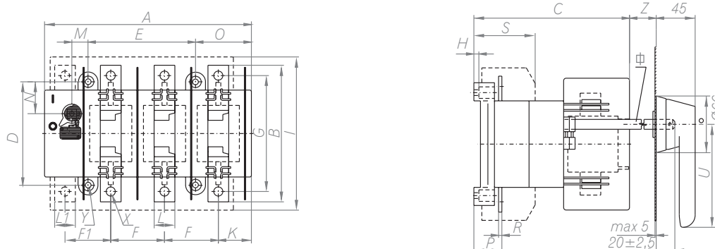
Rysunki wymiarowe RAB 00, RAB 1, RAB 2, RAB 3
