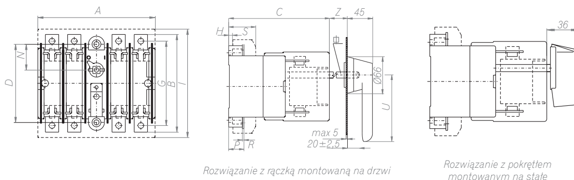
Rysunki wymiarowe RAB 000 (100 A)
