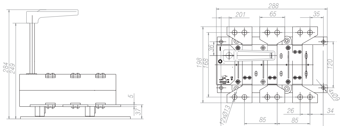
RIN 630/RA
